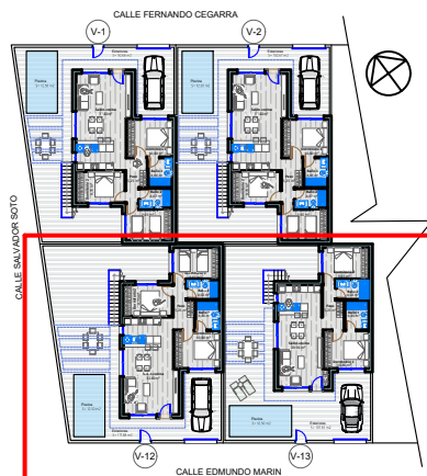
VIVIENDA TIPO 3 DORMITORIOS
